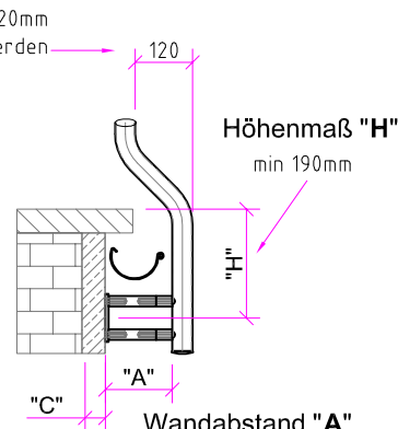
seitliche Montage gebogen um Regenrinne
