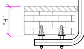
Montage unter Balkondecke
