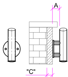
seitliche Montage
